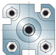
Profilo testate per alesaggio 20 End cup shape for bore 20
